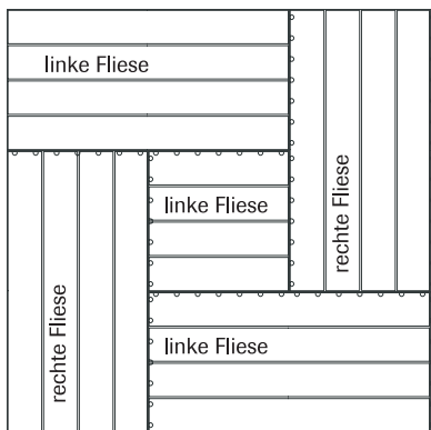
Beispiel Verlegemuster
